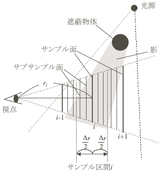
図3 サブサンプル面を用いたアンチエイリアシング。 Removing aliasing effects by using sub-sample planes.
